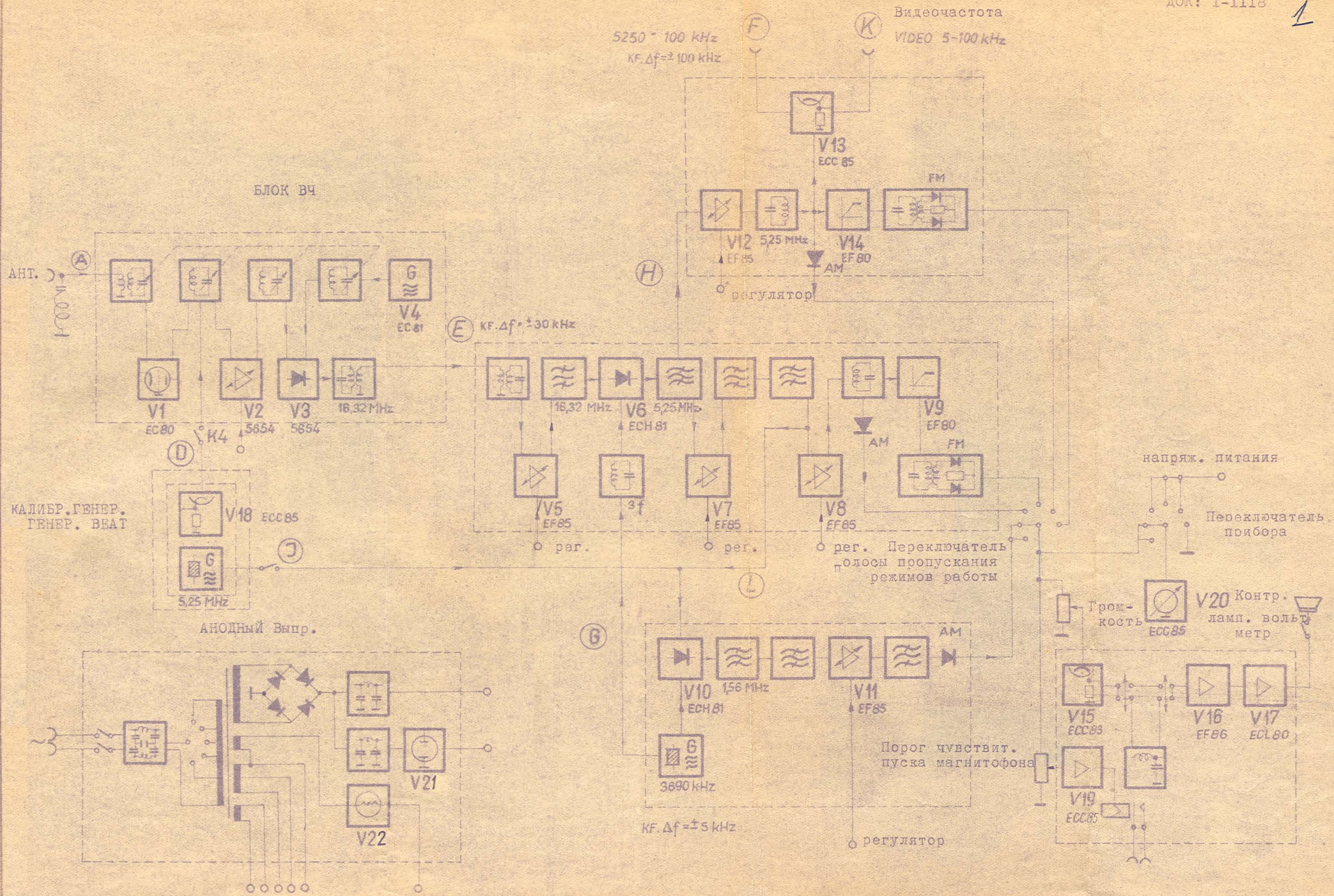
БЛОК-СХЕМА VU-21
